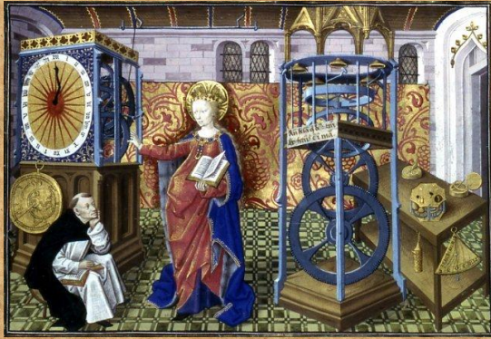
Mehanična ura.
